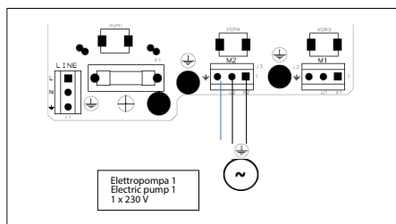
1 electrobomba
