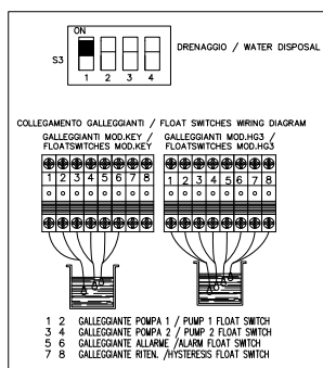
Drenaj 2 pompe
