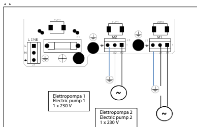
2 électropompes
