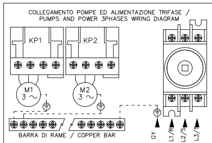
2 elektromos szivattyú
