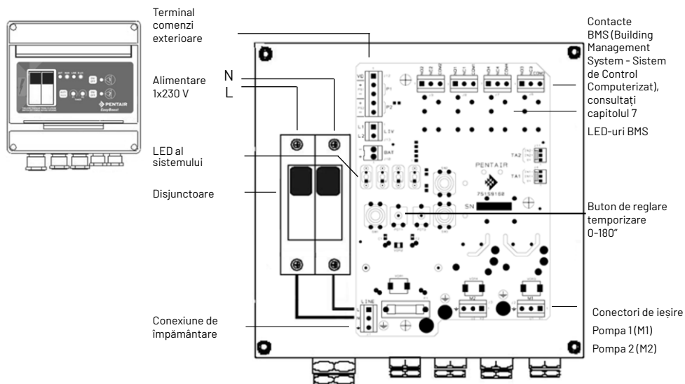
1 electropompă
