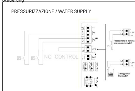
Wasserversorgung Zwei-Pumpen-Steuerung
