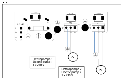
2 pompy elektryczne
