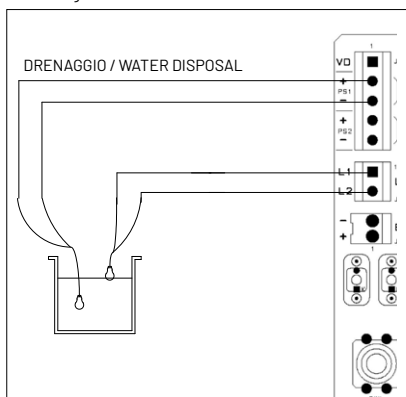
Wasserentsorgung Ein-Pumpen-Steuerung
