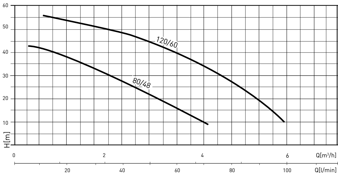
WYKRES PRACY POMPY
